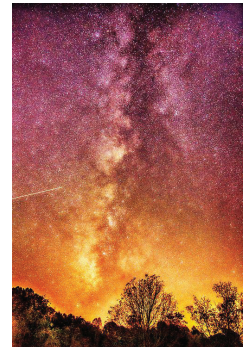
صورة مجرة التبانة
